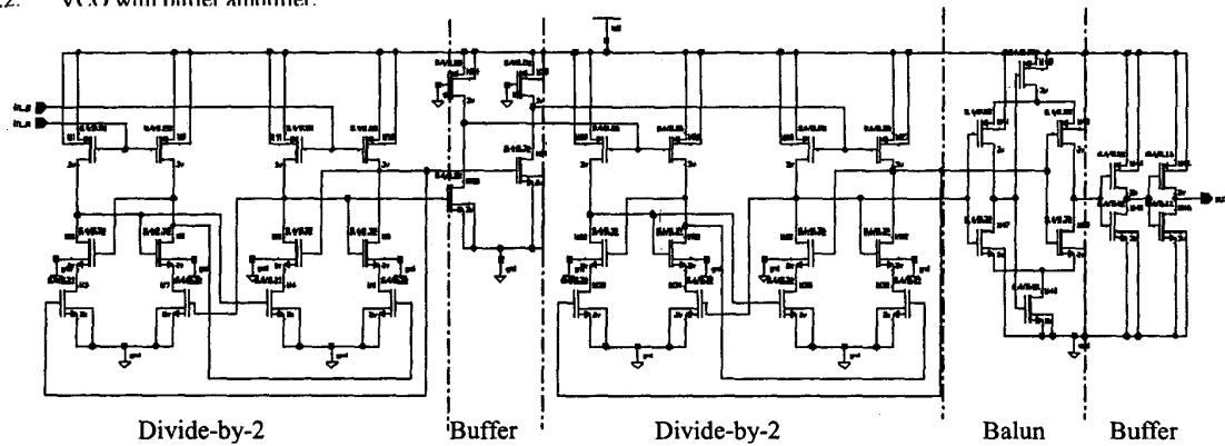
Fig. 3. Divide-by-4 circuit.
